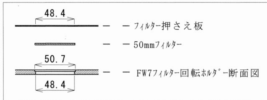
回転フォルダー
