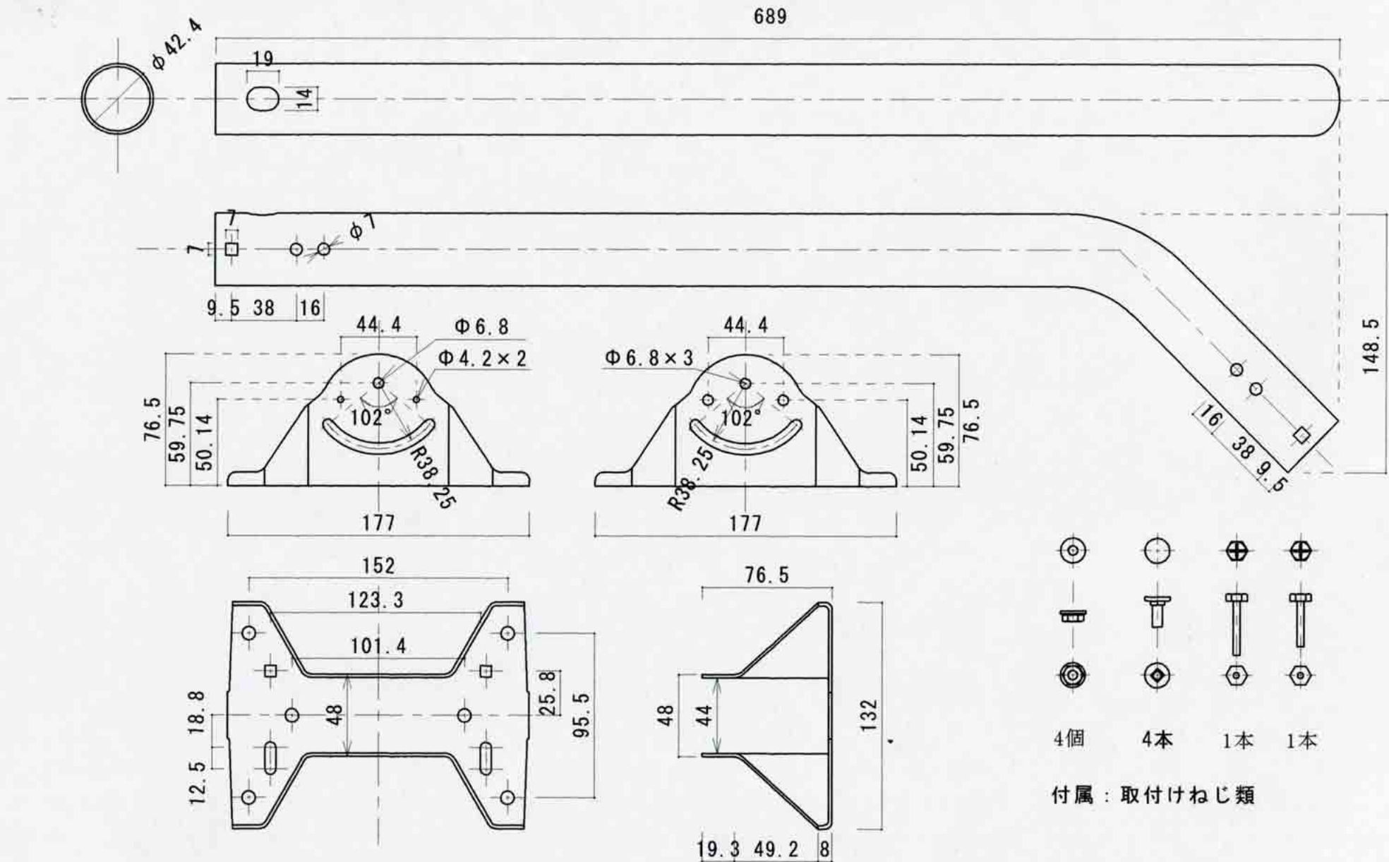
MGT aLL SKY CaM用28"ホールマウント金具
